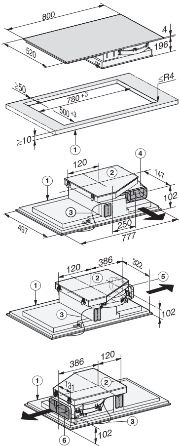
KMDA 7634 FL, KMDA 7476 FL (opbouw)
