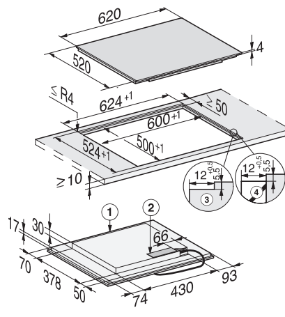
KM 7465 FL (vlakbouw)
