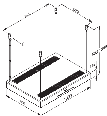
DA 6708 D eilanddampkap
