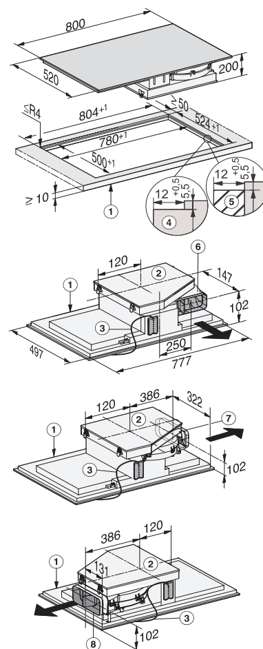
KMDA 7634 FL, KMDA 7476 FL (vlakbouw)
