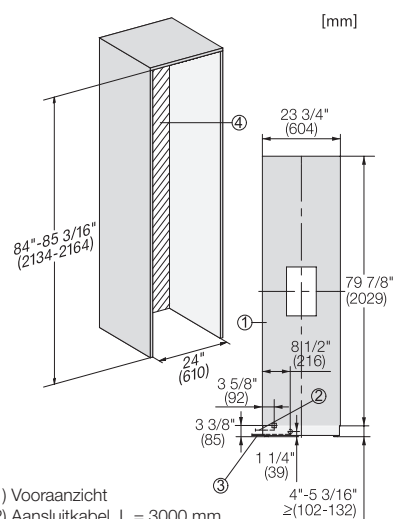
F 2672 Vi - aansluitingen
