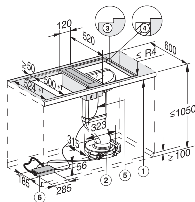
CSDA 7001 FL (vlakbouw)
