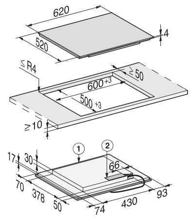
KM 7465 FL (opbouw)
