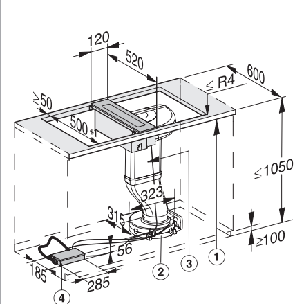
CSDA 7001 FL (opbouw)
