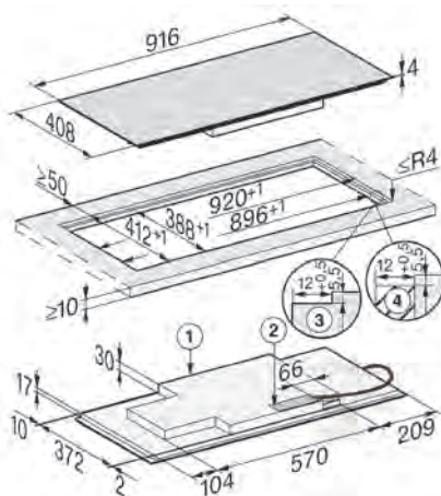
KM 7689 FL (vlakbouw)
