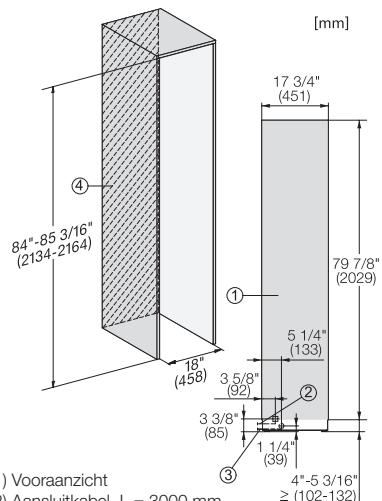
F 2412 Vi - aansluitingen
