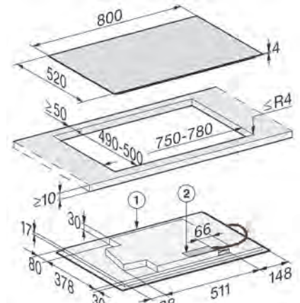
KM 7679 FL (opbouw)
