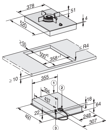
CS 7101-1 FL (opbouw)
