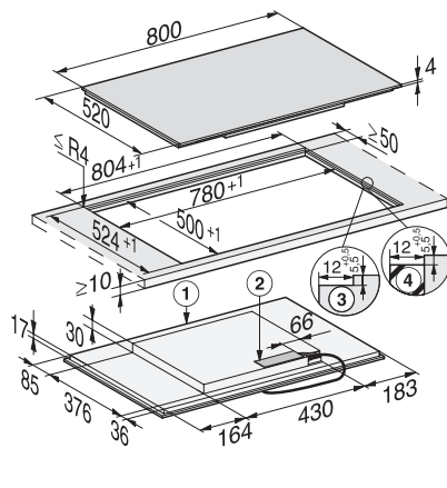
KM 7474 FL (vlakbouw)
