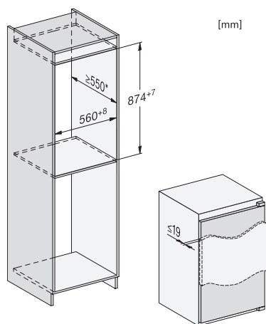
K 7113 F, K 7114 E, K 7113 D
