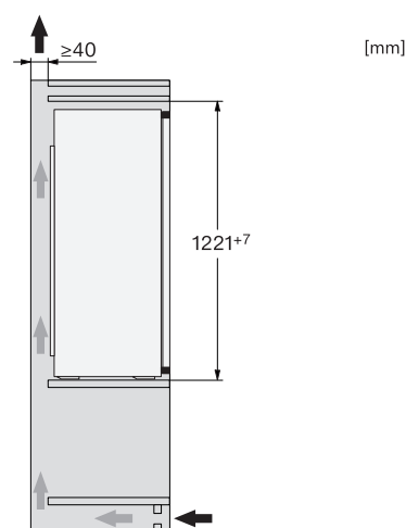
K 7313 F, K 7314 F, K 7313 D
