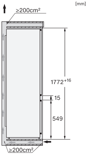
KF 7742 D, KF 7772 B
