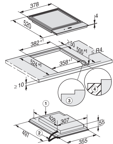
CS 7632 FL TeppanYaki (vlakbouw)
