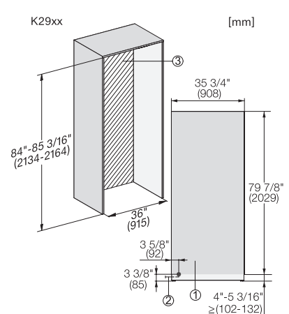
K 2902 Vi - aansluitingen
