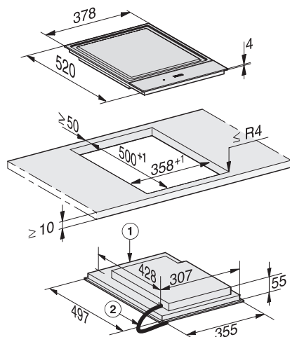
CS 7632 FL TeppanYaki (opbouw)
