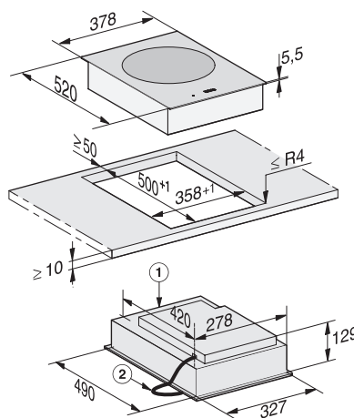
CS 7641 FL Wok (opbouw)
