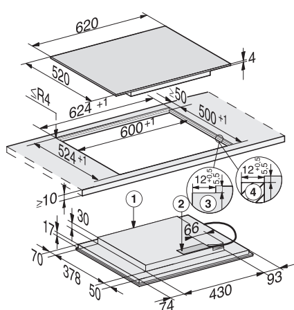
KM 7564 FL (vlakbouw)
