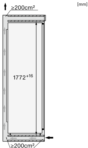
K 7733 E, K 7734 F, K 7743 E, K 7744 E, K 7763 E, K 7764 E, K 7773 D
