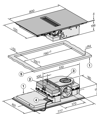
KMDA 7473 FLU (opbouw)
