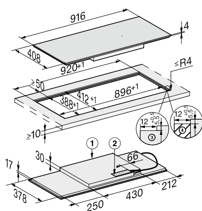
KM 7684 FL (vlakbouw)
