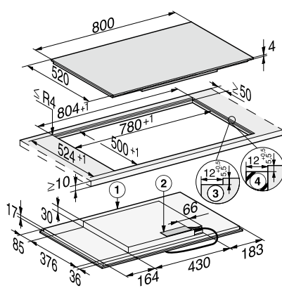
KM 7474 FL (vlakbouw)
