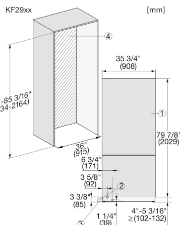
KF 2902 Vi, KF 2982 Vi - aansluitingen
