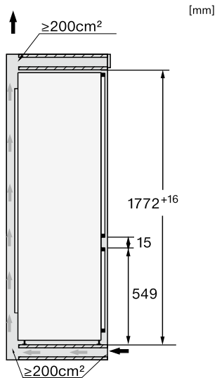
KF 7742 D, KF 7772 B
