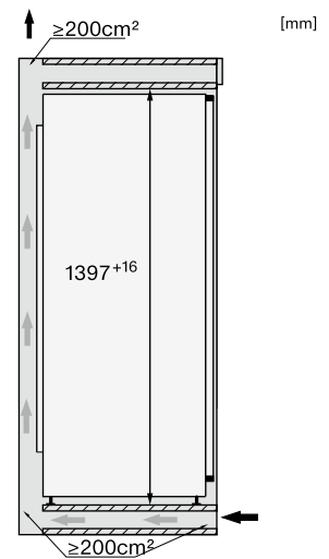
K 7433 E, K 7434 E, 7443 D, K 7444 D
