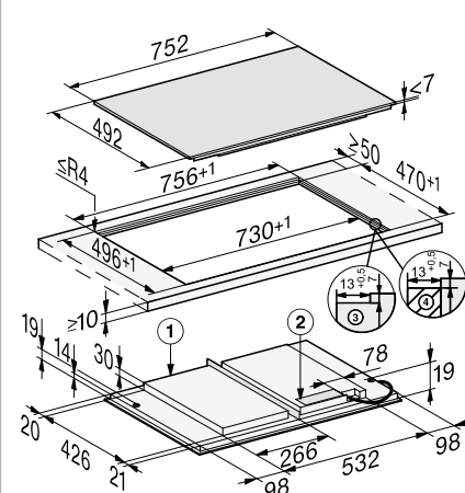
KM 7617 FX (vlakbouw)
