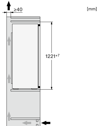
K 7313 F, K 7314 F, K 7313 D
