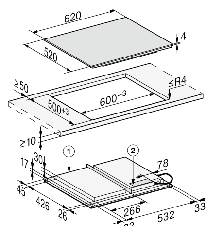
KM 7667 FL (opbouw)
