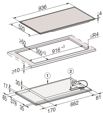
KM 7594 FL (opbouw)
