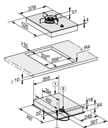
CS 7101-1 FL (opbouw)
