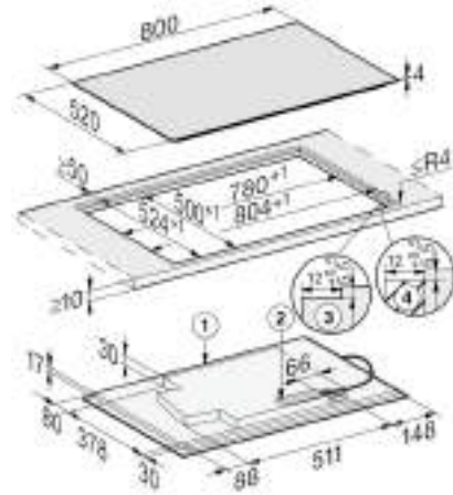
KM 7879 FL (vlakbouw)
