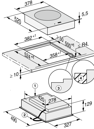
CS 7641 FL Wok (vlakbouw)
